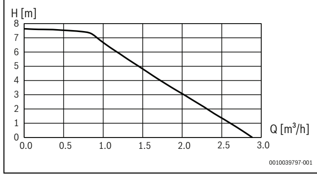
Res. 30 Birincil sirkülasyon pompası (PC0) kapasite eğrisi
