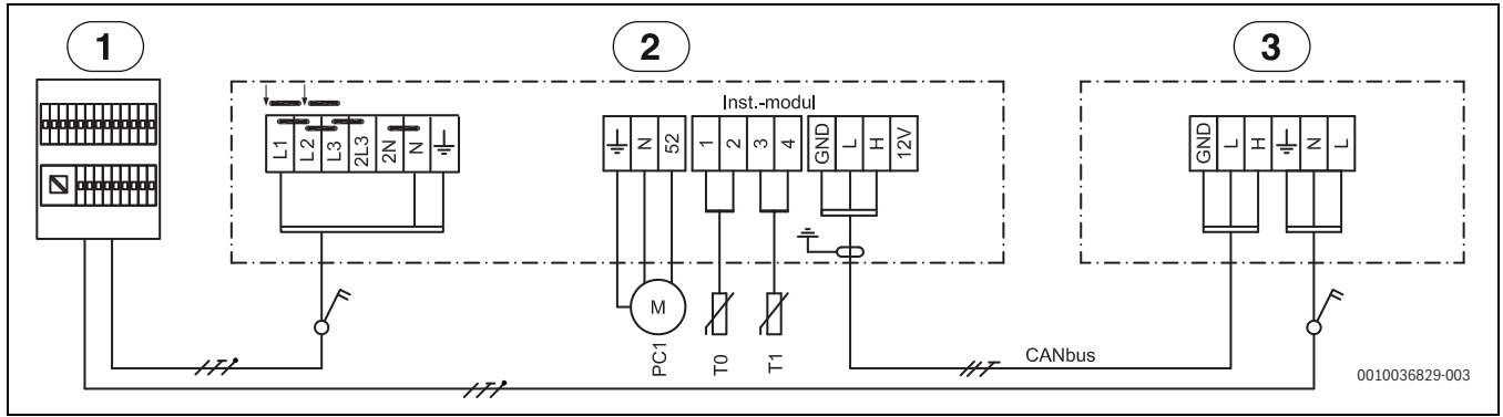
Res. 40 Devre şeması 5,85 kW 230 V~
