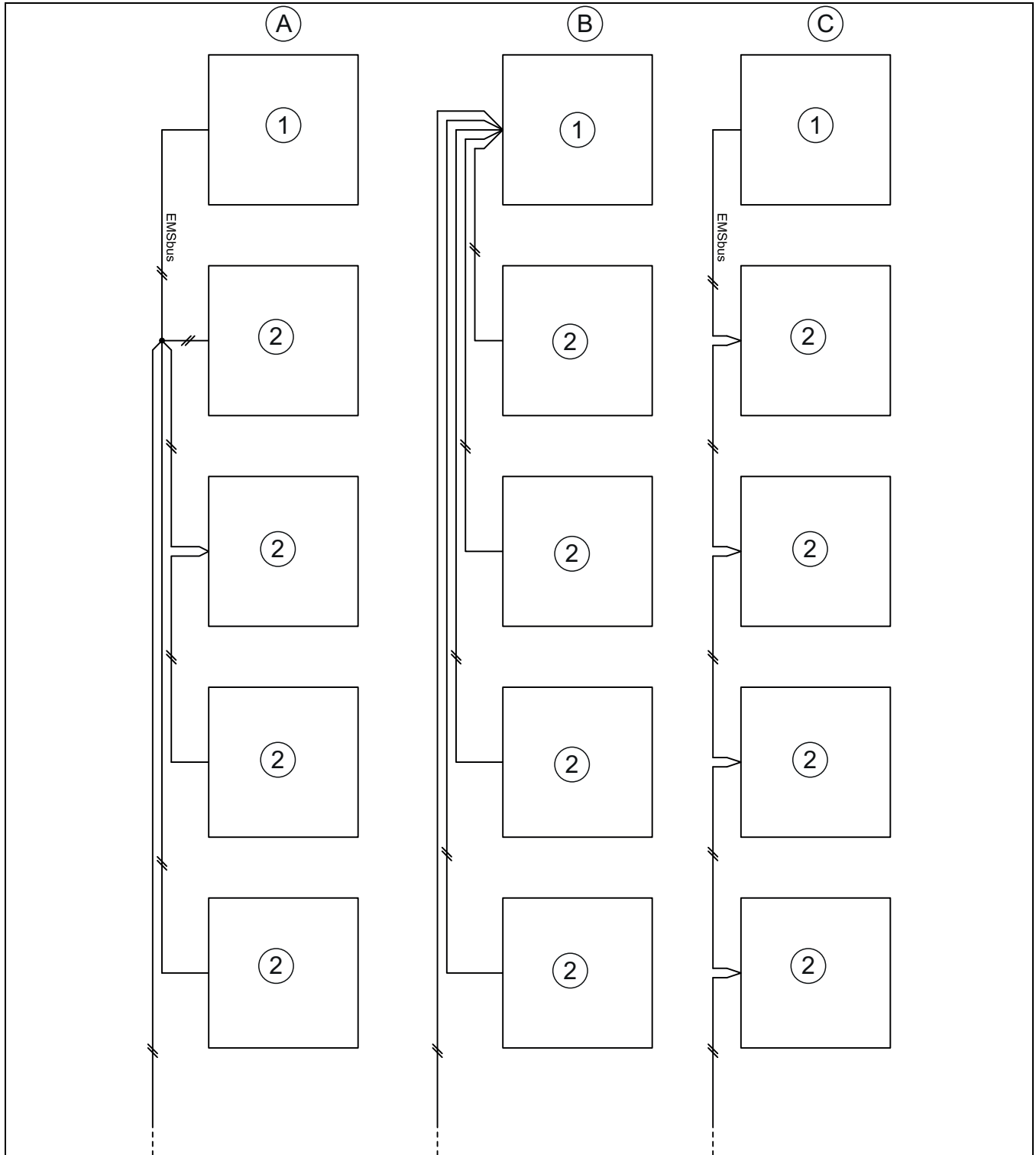
Res. 43 EMS-Bus için bağlantı seçenekleri
