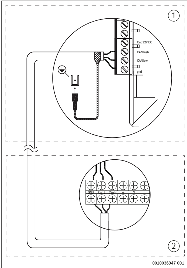
Res. 12 CAN-BUS bağlantısı
