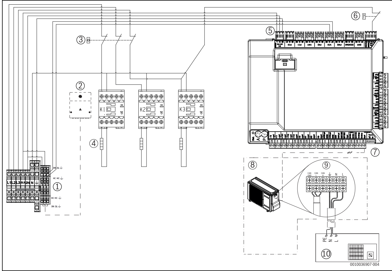
Res. 42 230V~ dış ünite ile 400 V 3 N~ iç ünite
