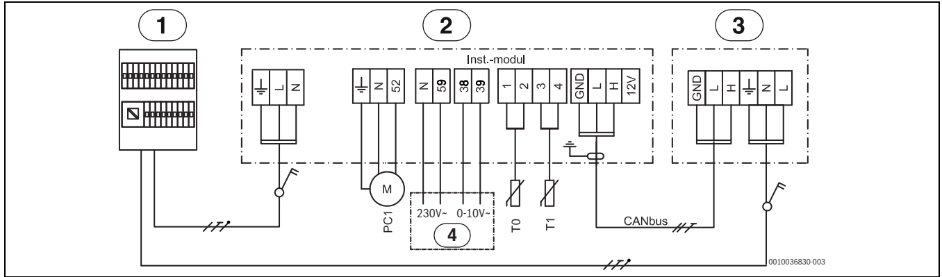
Res. 41 Devre şeması 5,85 kW 3 N~
