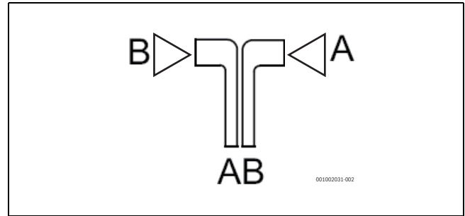
Res. 22 Dağıtıcı vana TW1 için hidrolik
