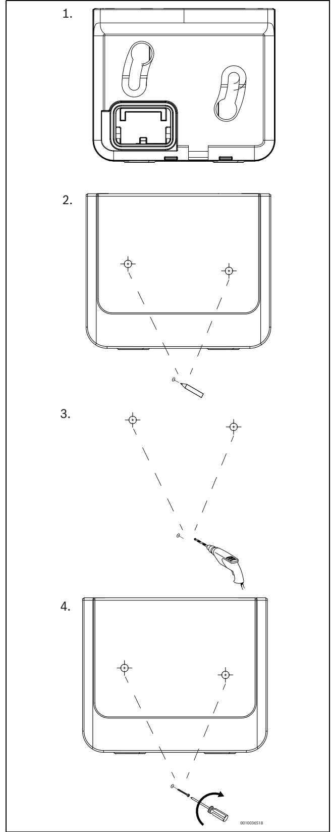
Res. 29 Tutucunun duvara montajı
