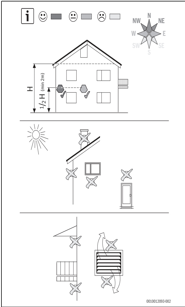
Res. 13 Dış hava sıcaklık sensörünün konumlandırılması
