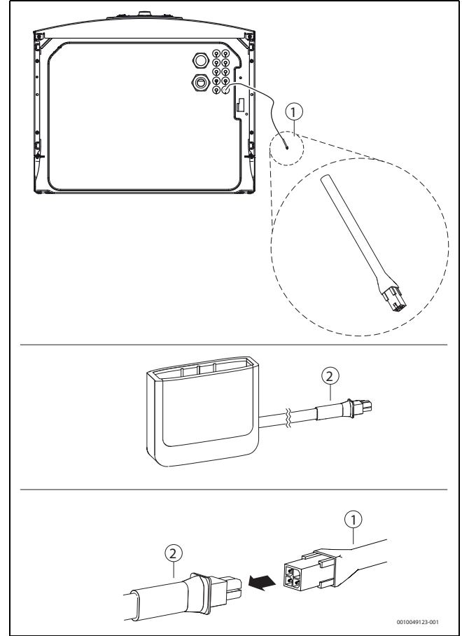
Res. 26 Connect-Key bağlantısını kurma.
