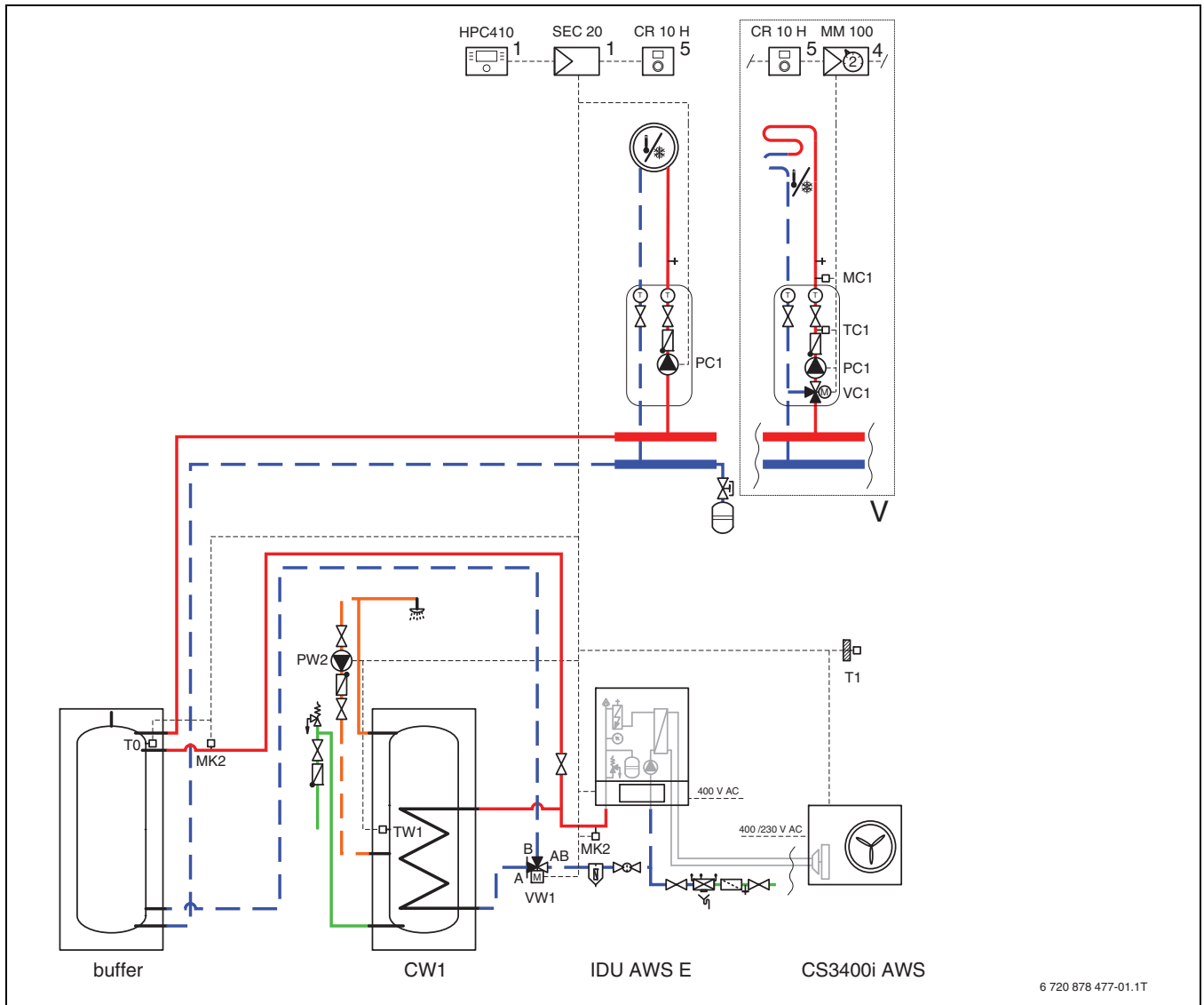
Res. 37 İç ünite ile dış ünite, depo ve bir veya daha fazla ısıtma devresi
