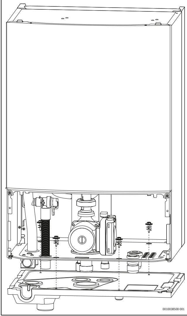
Res. 7 Toplama kabının monte edilmesi
