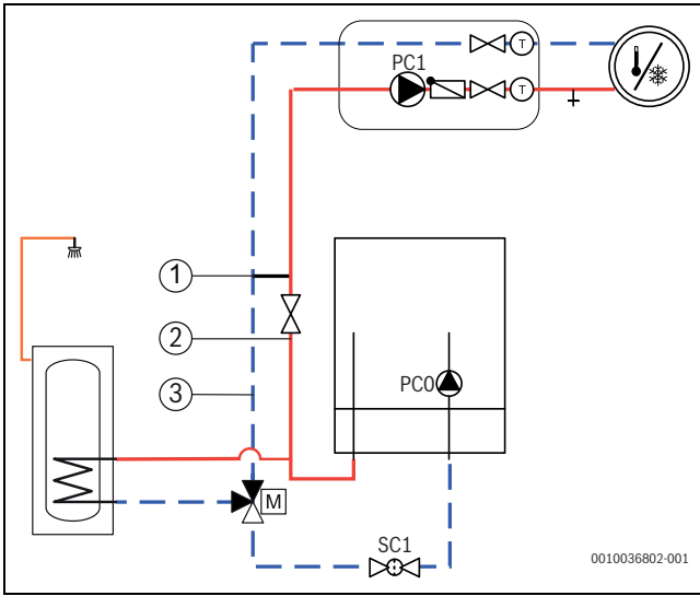
Res. 32 İç ünite ısıtma devresi ve kullanım suyu hazırlama
