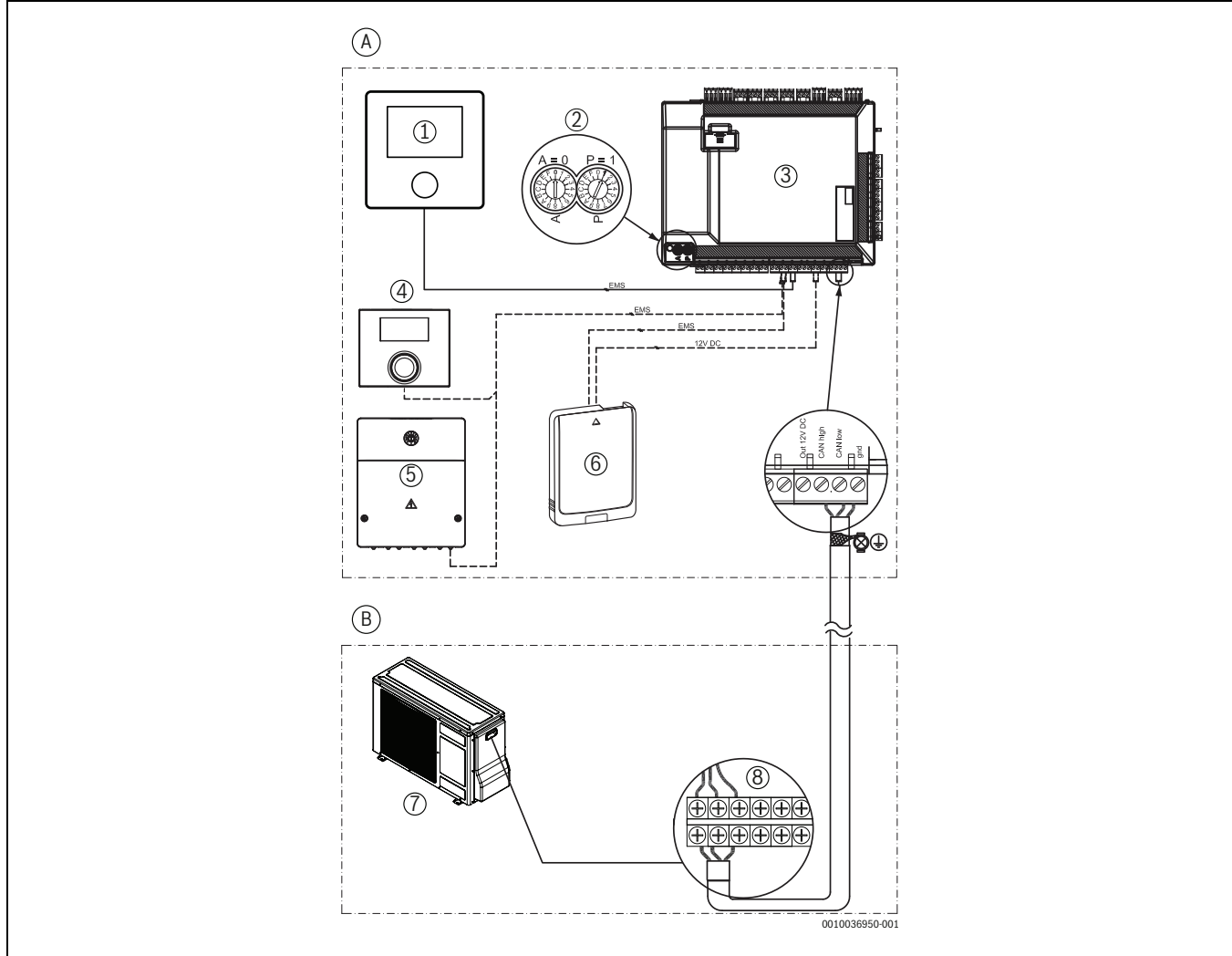
Res. 39 CAN ve EMS bağlantıları
