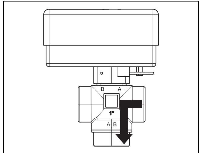
Res. 23 Temas kapalı, bağlantı A açık
