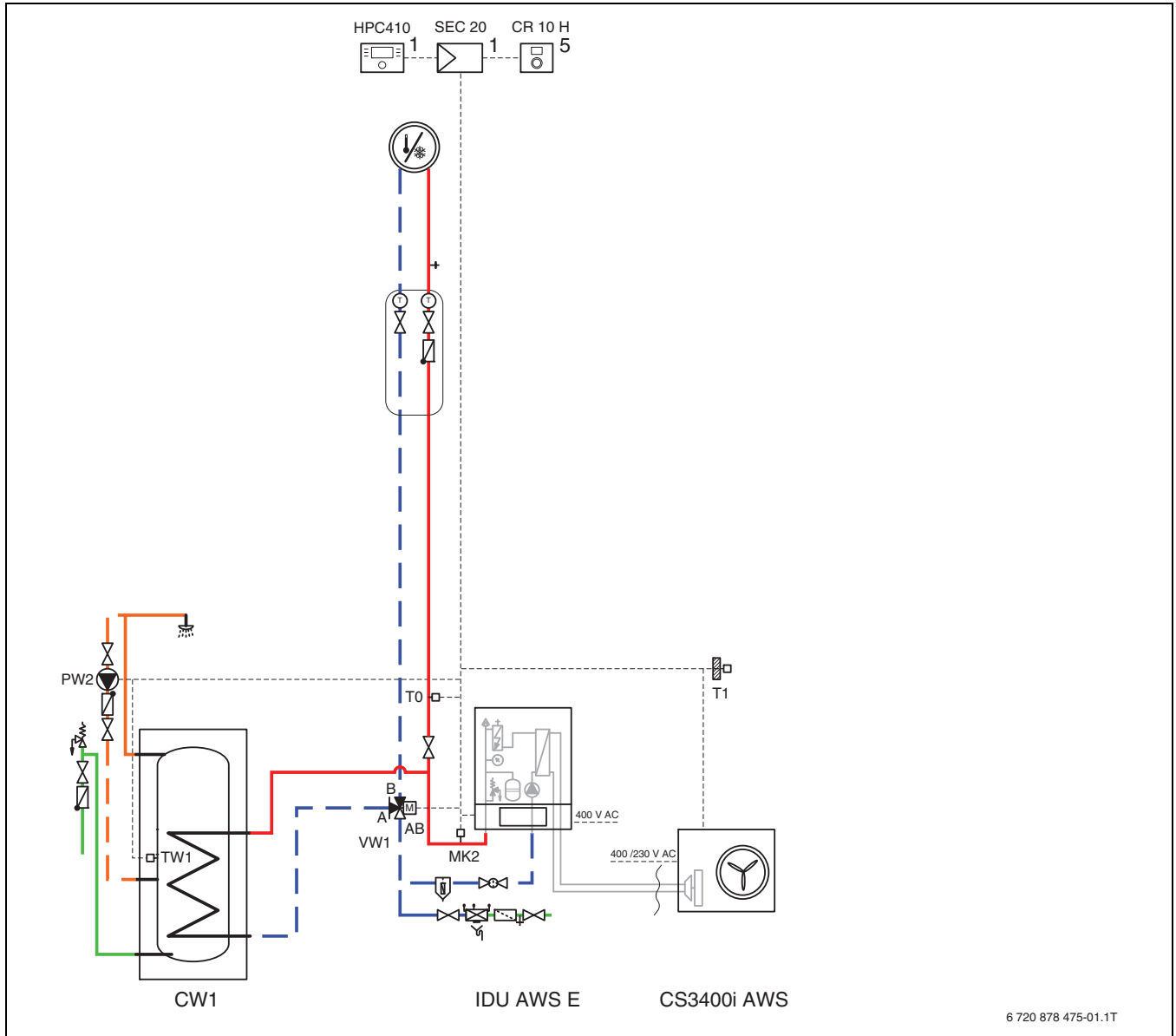
Res. 35 İç ünite ile dış ünite ve bir ısıtma devresi
