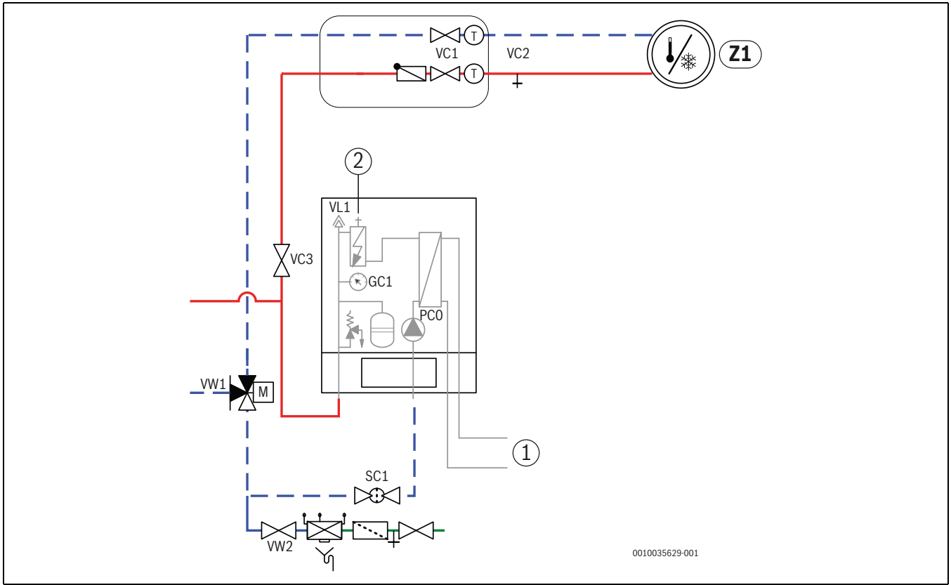
Res. 9 Entegre elektrikli ısıtıcılı ve ısıtma sistemli iç ünite
