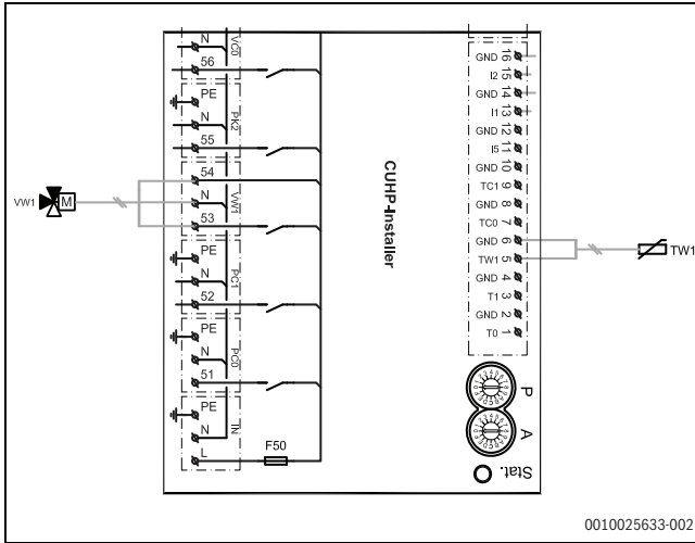
Res. 20 Montaj devre kartında dağıtıcı vana VW1 bağlantısı
