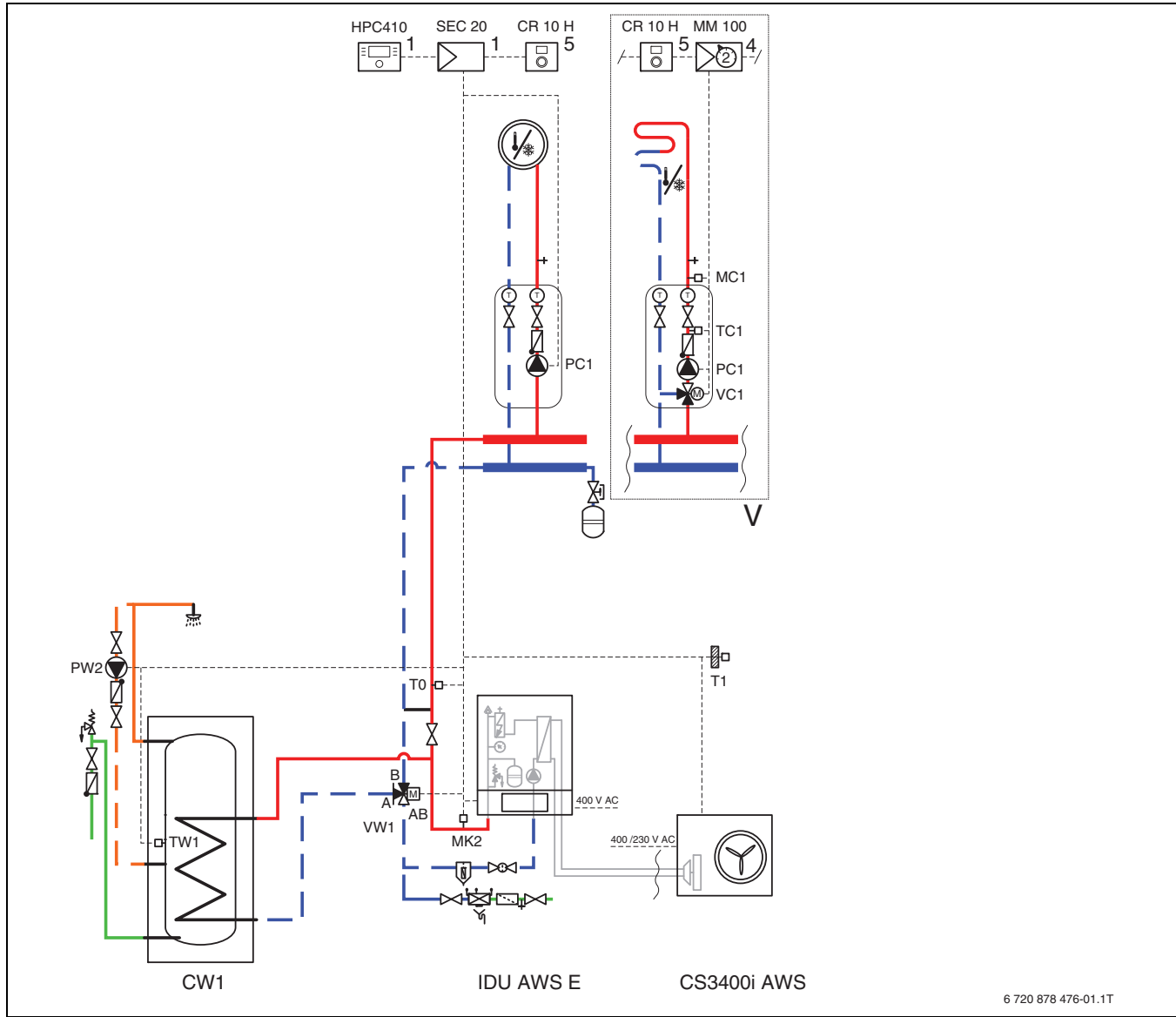
Res. 36 İç ünite ile dış ünite, sıcak kullanım suyu ve bir veya daha fazla ısıtma devresi
