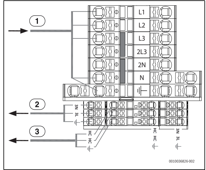
Res. 14 Elektrik bağlantı klemensleri, 5,85 kW 400 V 3 N~
