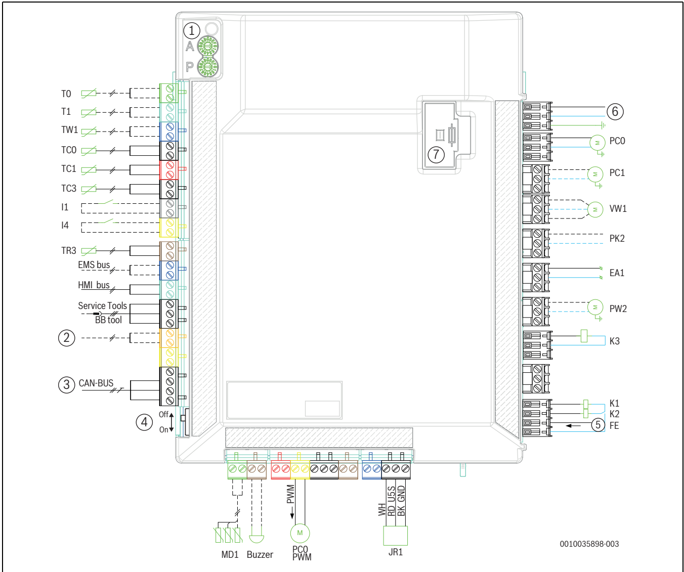
Res. 38 İç ünite montaj devre kartı
