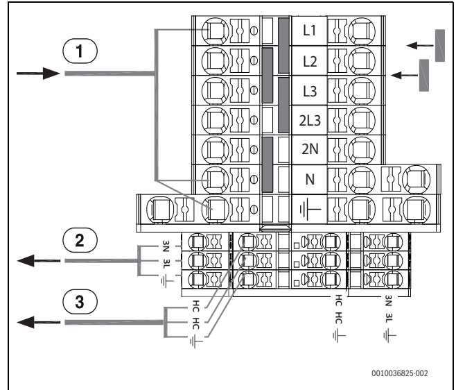
Res. 15 Elektrik bağlantı klemensleri, 5,85 kW 230 V
