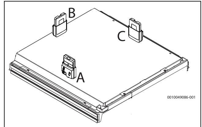
Res. 27 Tutucunun iç ünitenin üst parçasına takılması. Şekilde tutucuya ek olarak tutucu içinde oturan Connect-Key gösterilmektedir
