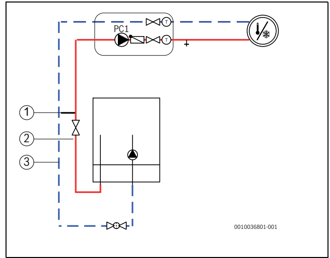
Res. 31 Isıtma devreli ve baypaslı iç ünite
