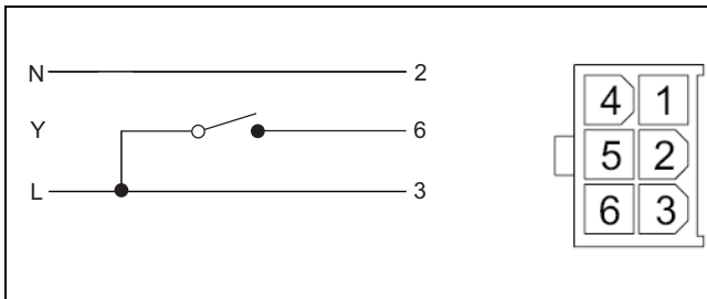
Res. 21 Molex fişi
